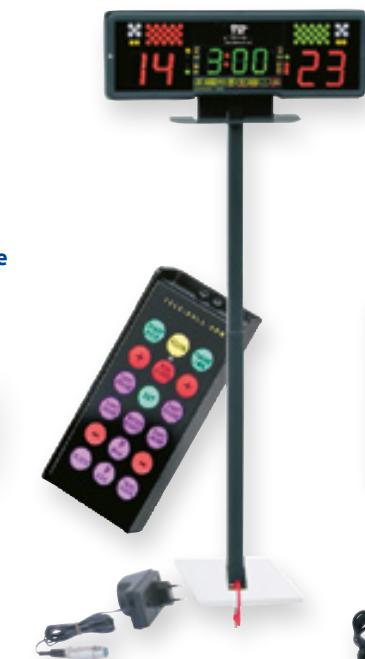
45FA5 Officially approved FIE 3-weapon scoring machine with remote control and power supply OR IN SET Tőr, párbajtőr, kard kijelző, FIE, távirányítóval és adapterrel, vagy szettben
